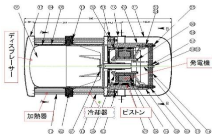
新型フリーピストンSE設計図(計画中) (サーモ技研(株))
