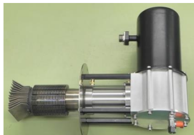
MOMOSEエンジン 200W (株)ジェー.ピー.イー
