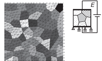
図2 解析モデルの要素分割(左)と負荷条件(右)
