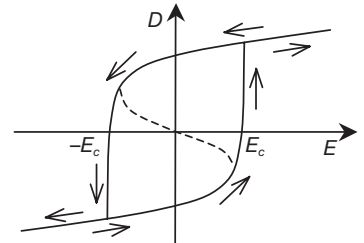
図1 材料非線形性 (電気変位 D -電界 E 履歴)
